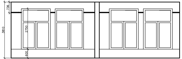
СЕЧЕНИЕ 1 - 1
