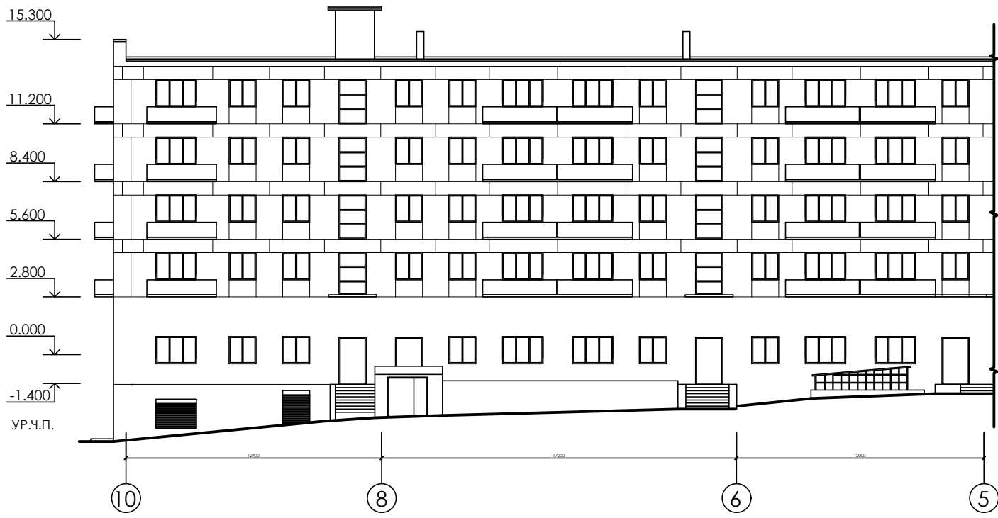
ФАСАД 10 - 1
