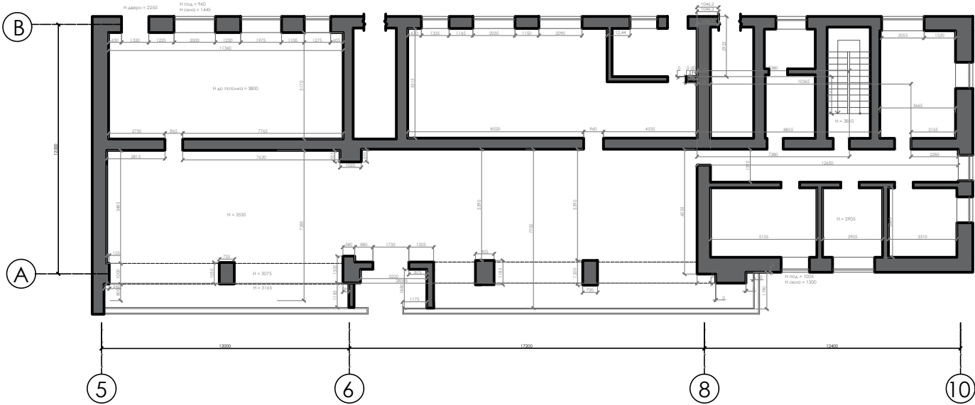
ПЛАН 1 ЭТАЖА
