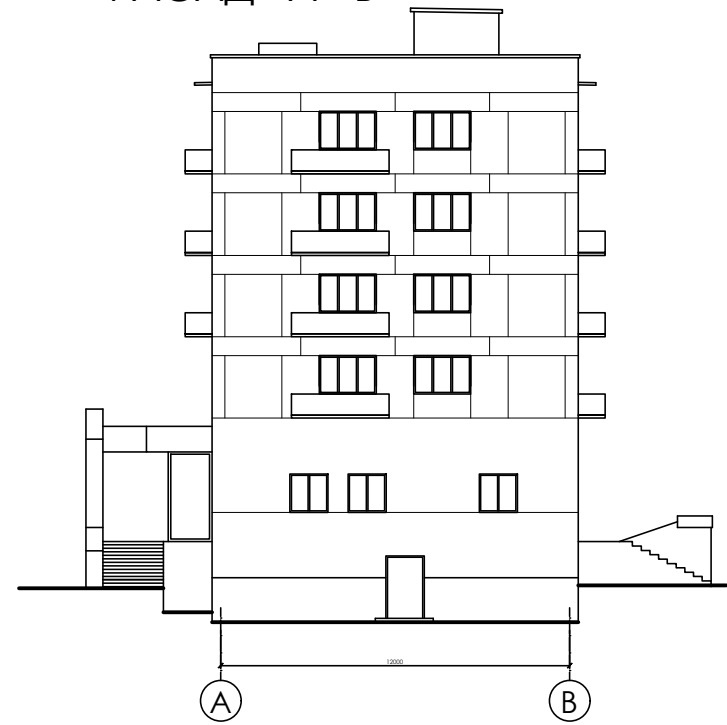
ФАСАД А - В
